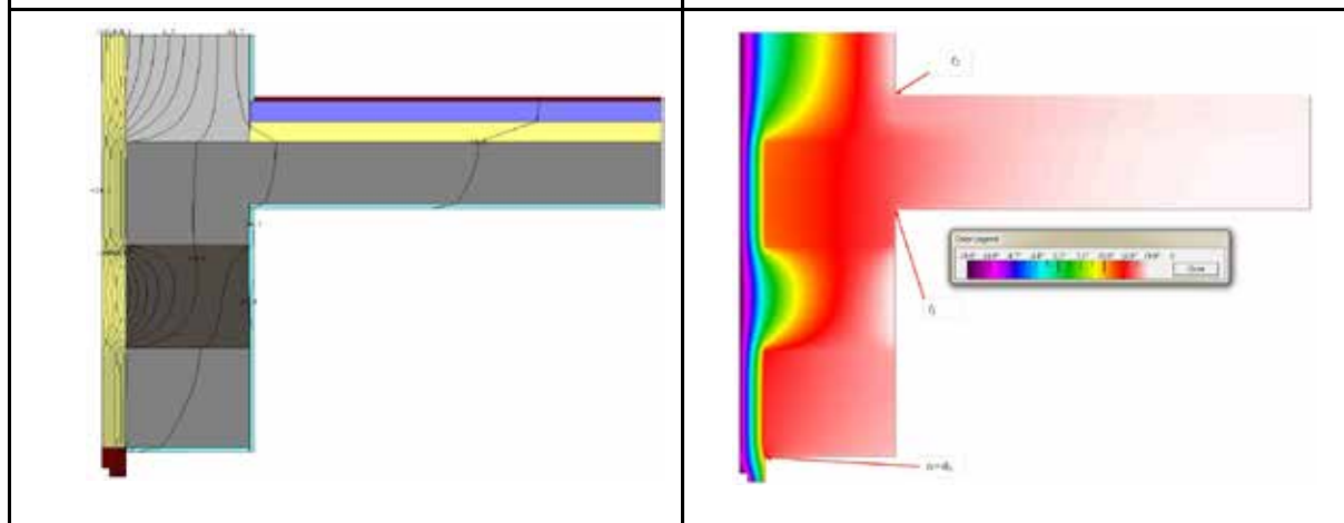
Rys. M11.1. Pole temperatur w przekroju. Izolinie i pole temperatury w skali barw.
