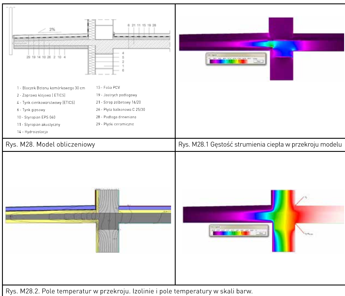
Tablica 6.28. Obliczone parametry ciepłno-wilgotnościowe węzła.
