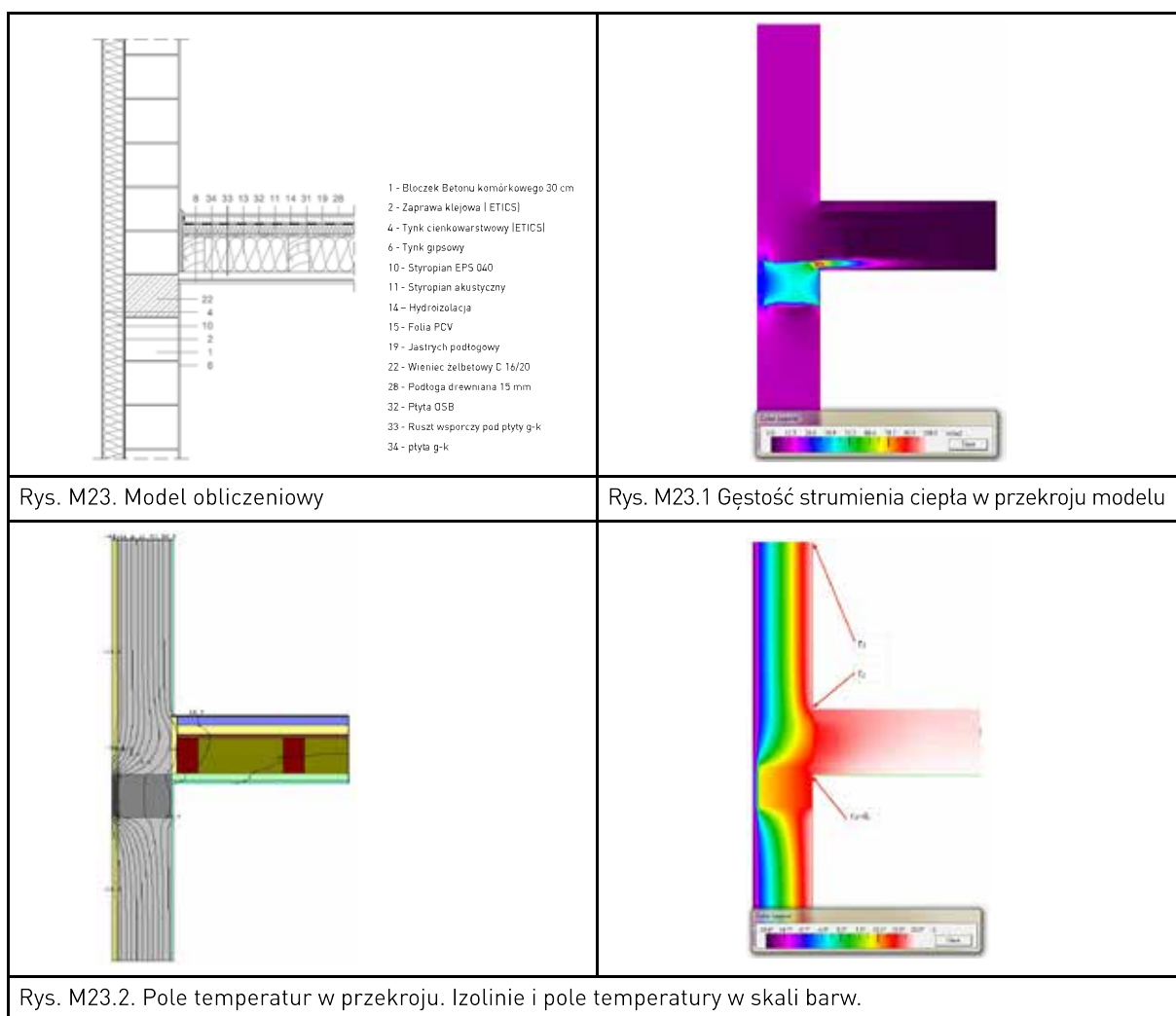
Tablica 6.23. Obliczone parametry ciepłno-wilgotnościowe węzła.
