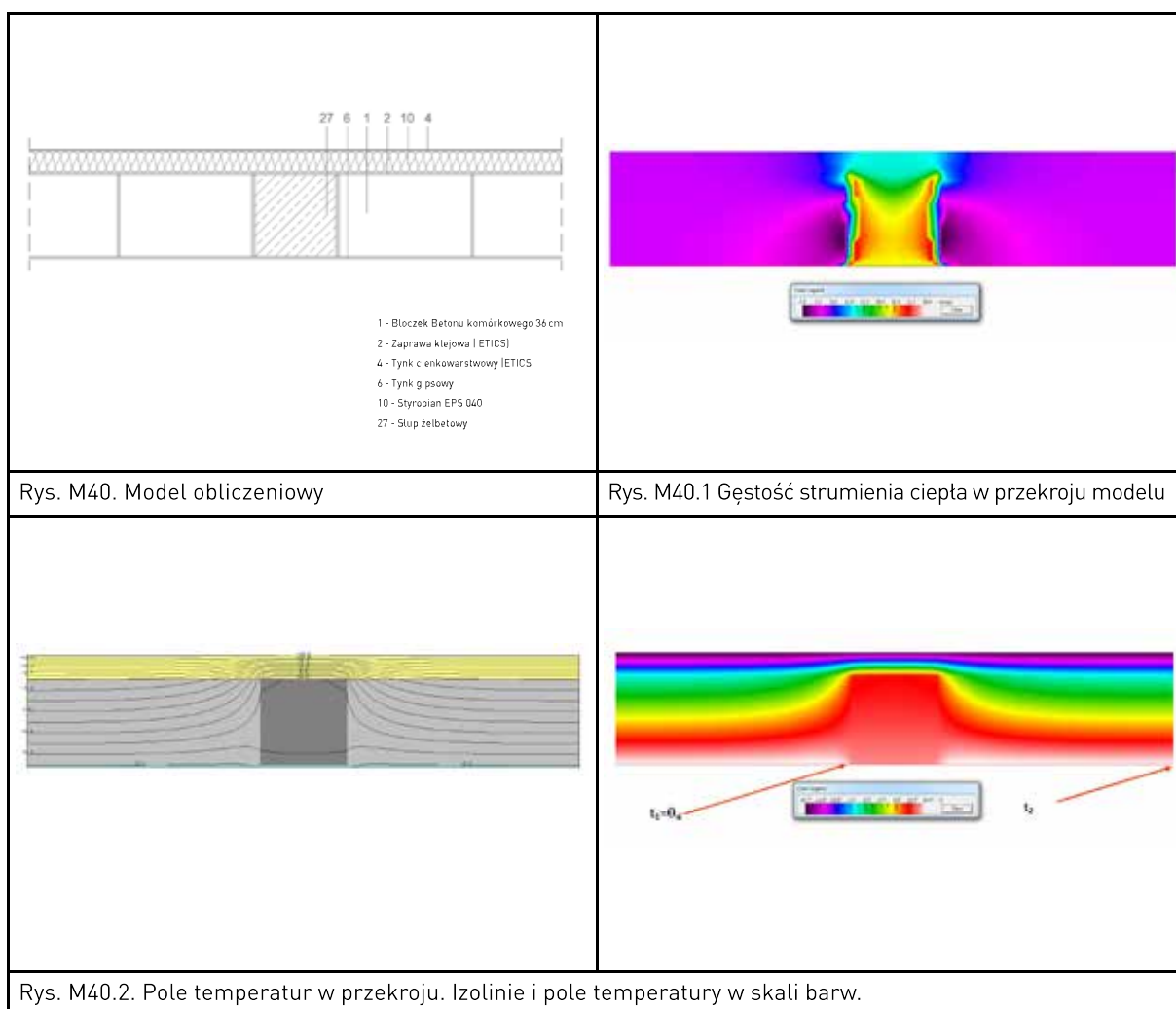
Tablica 6.40. Obliczone parametry ciepłno-wilgotnościowe węzła.
