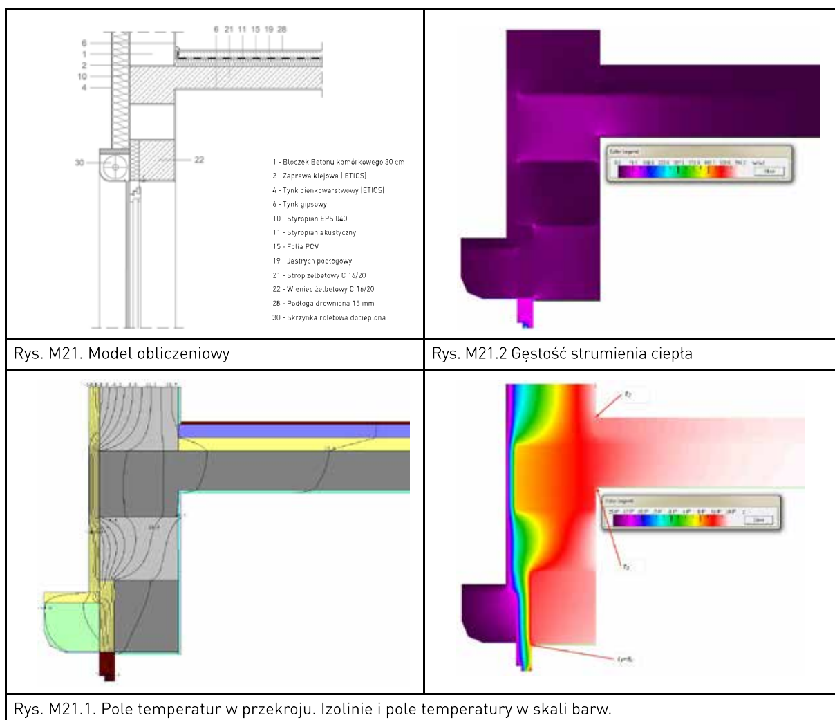
Tablica 6.21. Obliczone parametry ciepno-wilgotnościowe węzła.
