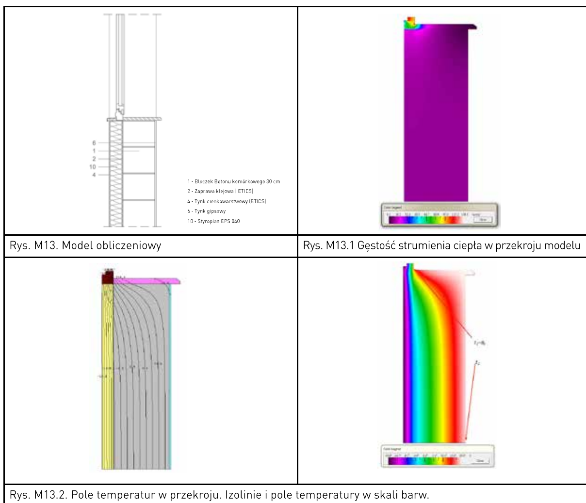
Tablica 6.13. Obliczone parametry ciepłno-wilgotnościowe węzła.
