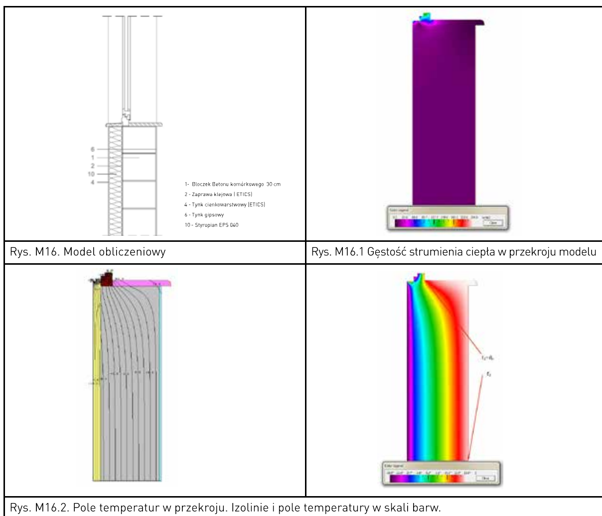
Tablica 6.16. Obliczone parametry cieplno-wilgotnościowe węzła.
