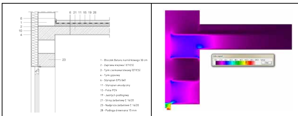
Rys. M11. Model obliczeniowy
