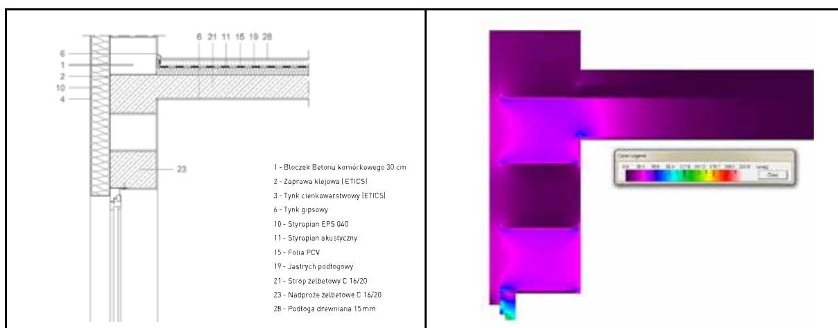
Rys. M14. Model obliczeniowy
