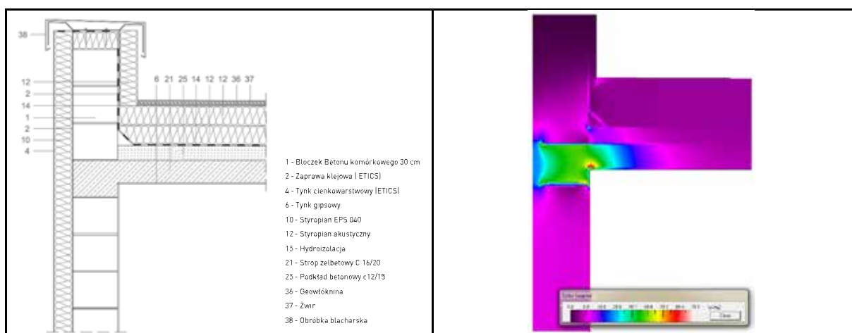
Rys. M32. Model obliczeniowy
