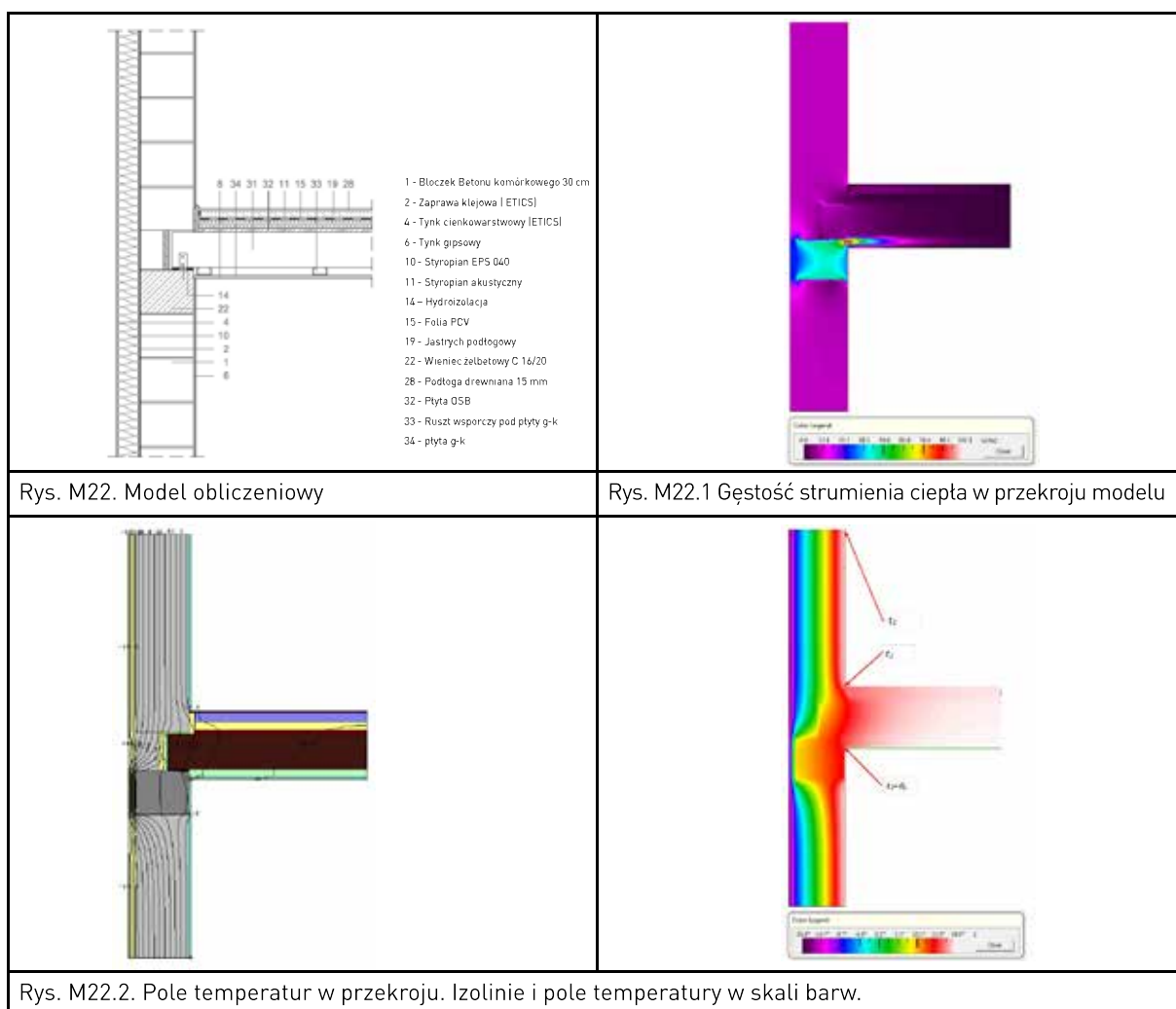
Tablica 6.22. Obliczone parametry cieplno-wilgotnościowe węzła.
