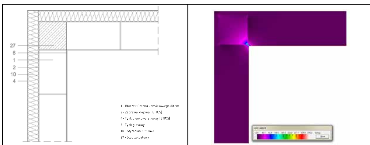
Rys. M36. Model obliczeniowy
