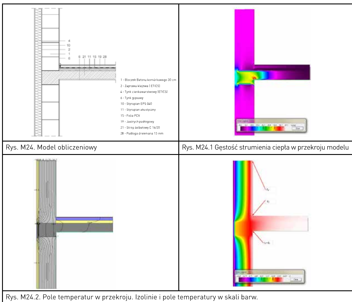
Tablica 6.24. Obliczone parametry cieplno-wilgotnościowe węzła.
