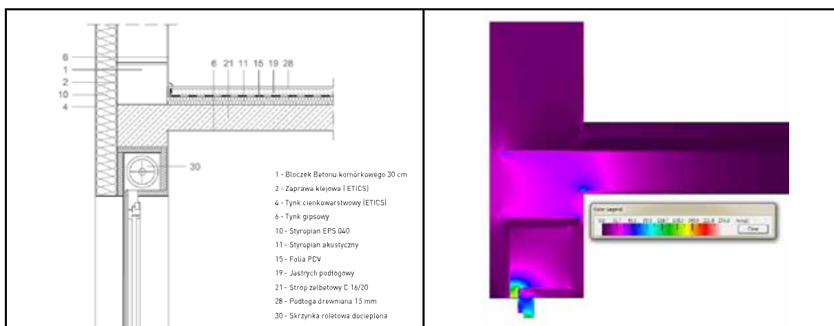
Rys. M20. Model obliczeniowy
